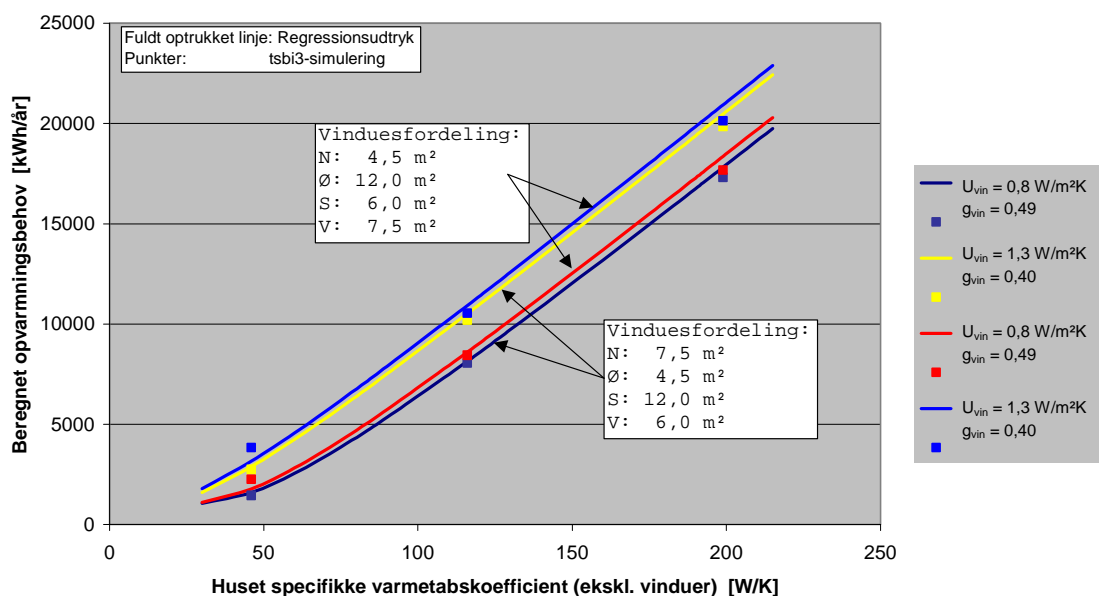
Figur 15. Sammenligning mellem resultatet af tsbi3 simuleringer og resultat af regressionsudtryk. Kurver og punkter med samme farve er samhörrende.
