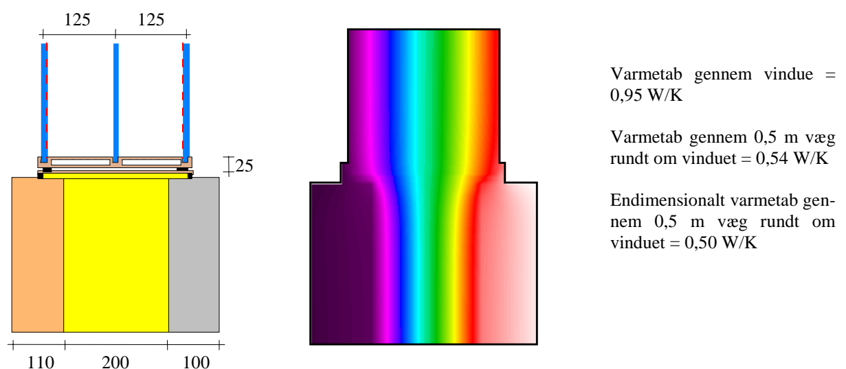
Figur 28. Eksempel på vindue tilpasset væggen's isoleringstykkelser. Resultat fra projektet ”Vinduer med smal ramme/karmkonstruktion og stort lys- og solindfald” [11].
